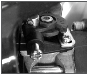
Рис. 16 Винт настройки оборотов холостого хода
