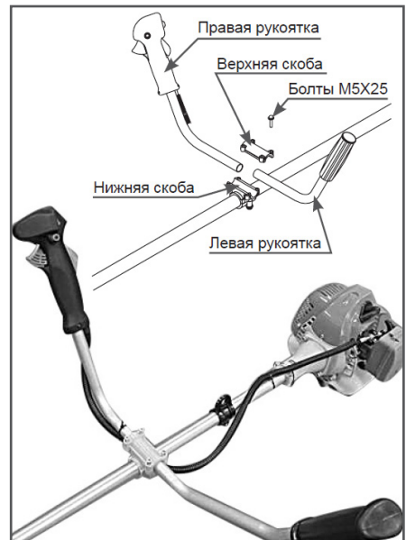
Рис. 4 Установка рабочей ручьятки
