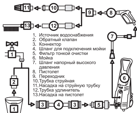
Рис. 12 Схема подключения аппарата моющего высокого давления с дополнительным оборудованием
