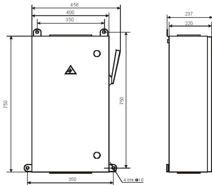
Рис. 1. Внешний вид, габаритные и установочные размеры корпуса ящика силового ЯРП-400-Узола.
