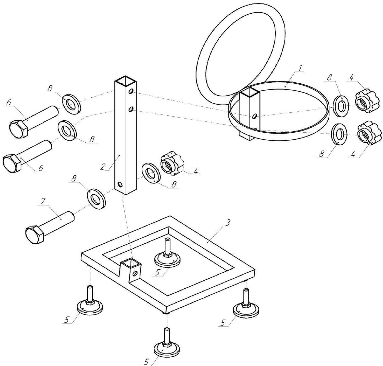
Спецификация на стойку для мусорных мешков 1 корзина
